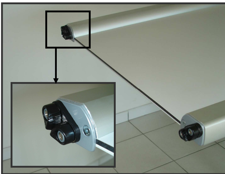
Les attaches liens en tête des profilés du panneau de table
